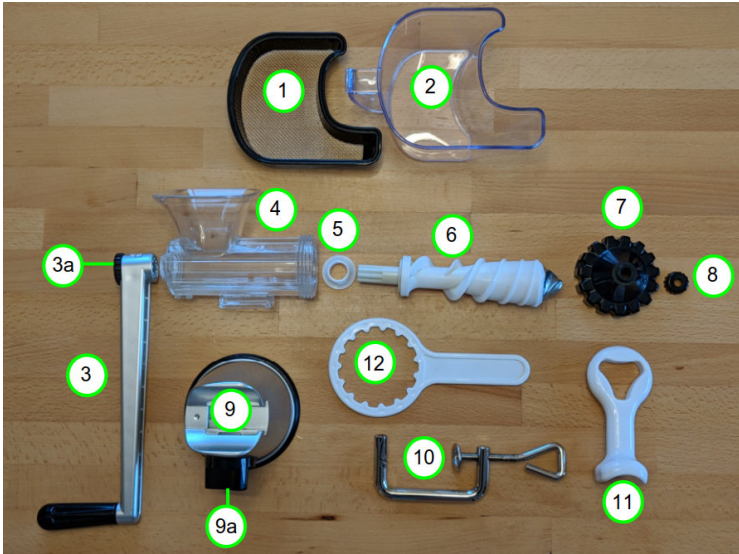
Zusammenbauen Bauteile Nummer 3, 4, 5, 6, 7, 8
