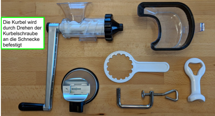
Zusammenbauen Bauteile Nummer 3, 4, 5, 6, 7, 8
